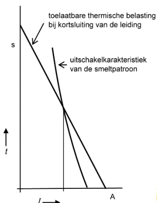
Figuur 3 – Het verband tussen de uitschakelkarakteristiek van de smeltpatroon en de toelaatbare thermische belasting bij kortsluiting van de leiding
