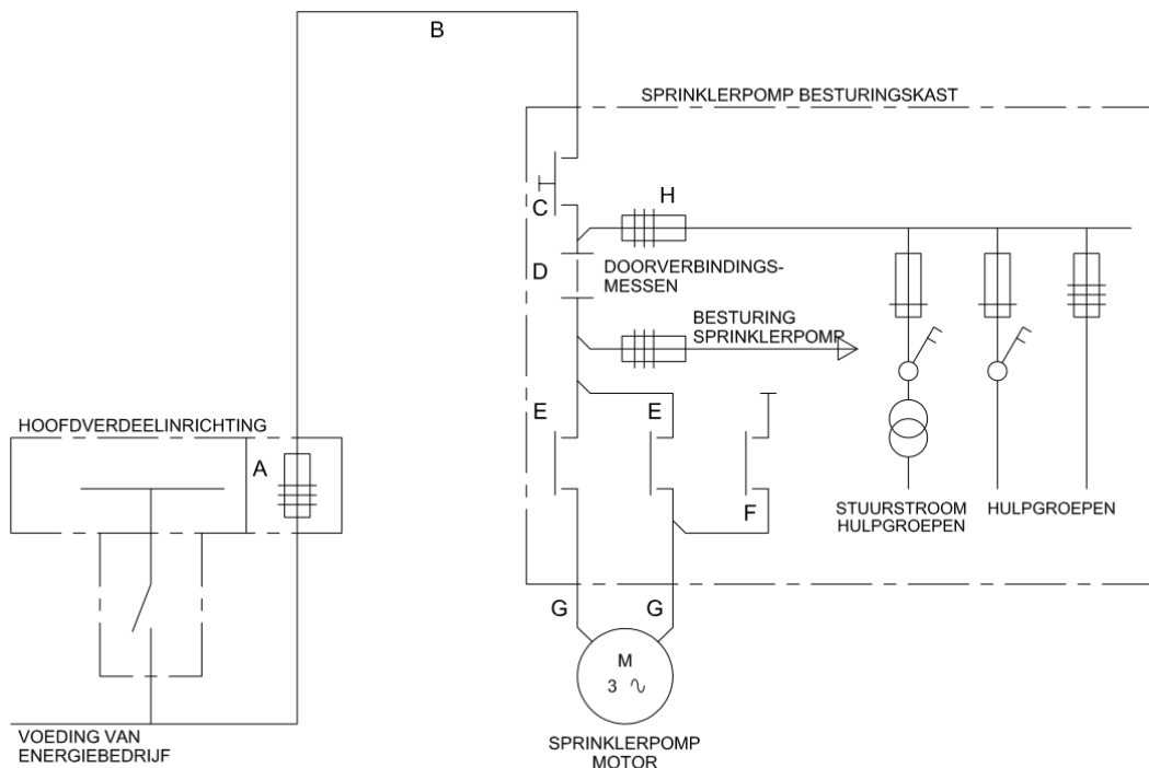
Figuur 1 - Schema sprinklerpomp zonder onderbeveiliging.
