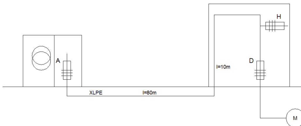
Figuur 7 - Situatieschets
