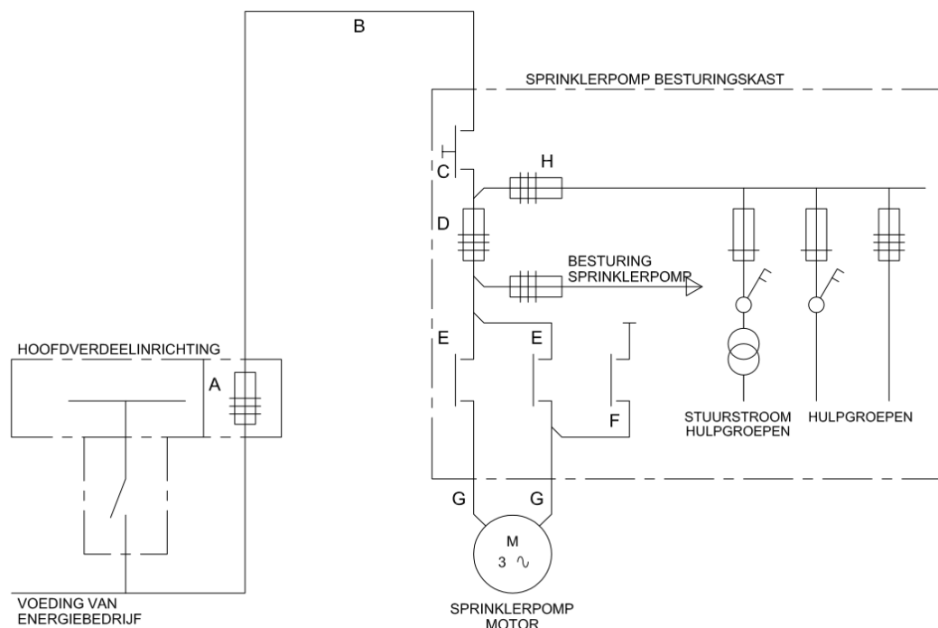
Figuur 2 - Schema sprinklerpomp met onderbeveiliging.
