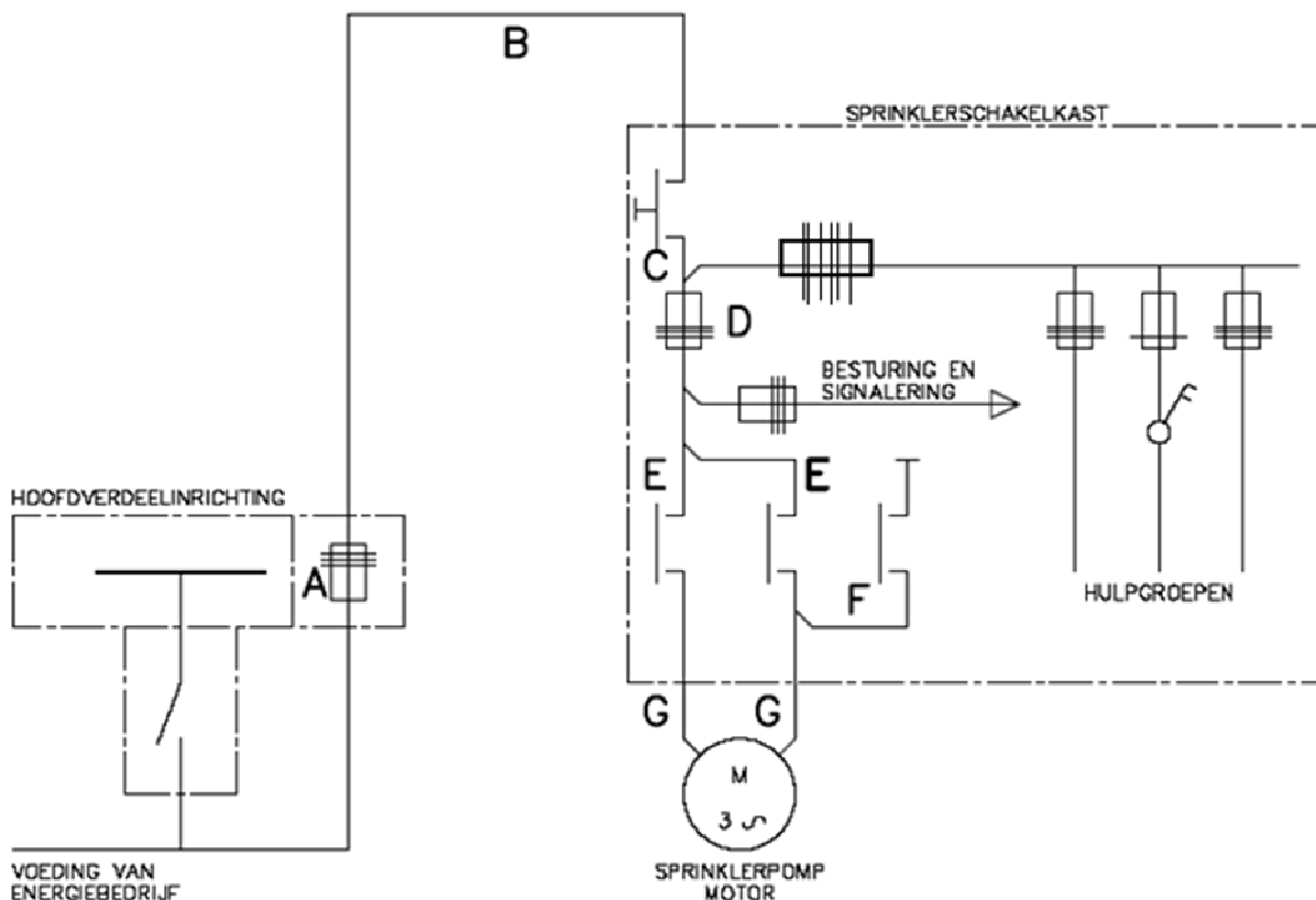
Figuur 2 - Schema sprinklerpomp met onderbeveiliging.
