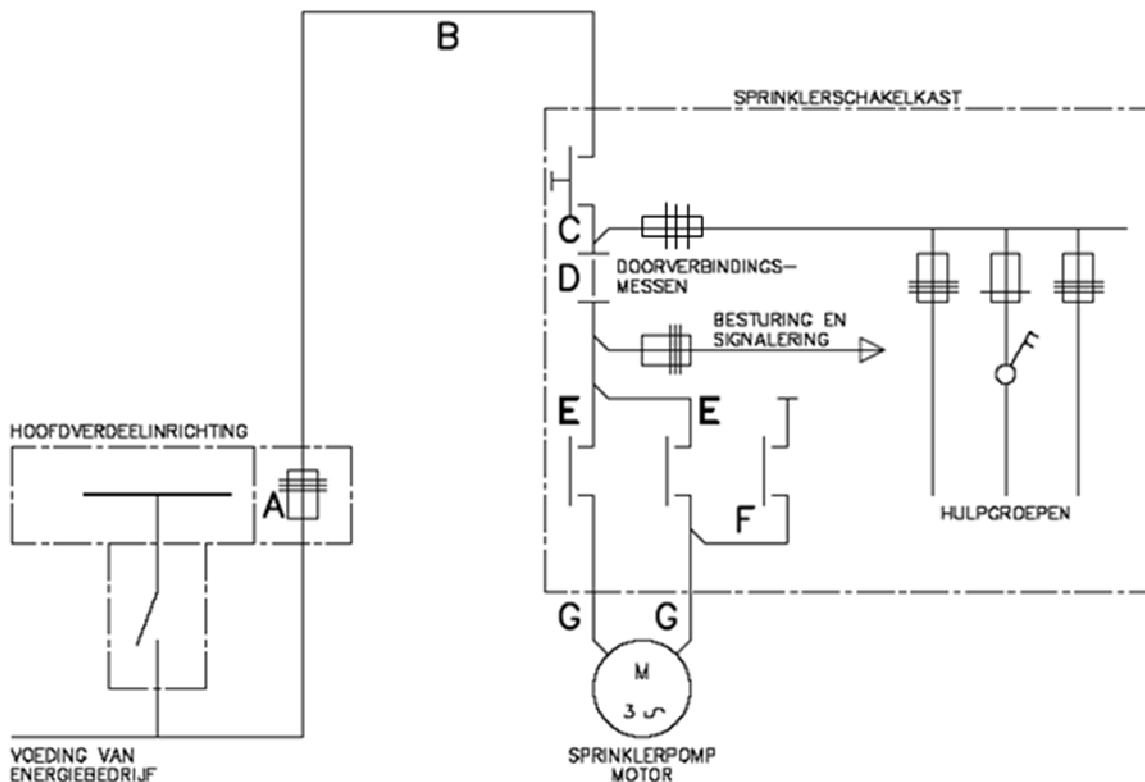
Figuur 1 - Schema sprinklerpomp zonder onderbeveiliging.
